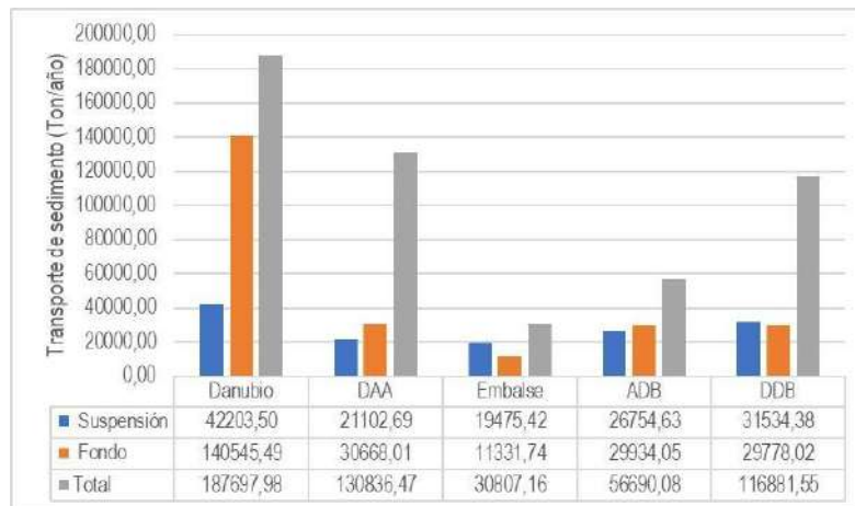
Figura 4 Transporte de sedimentos (Ton/año).
