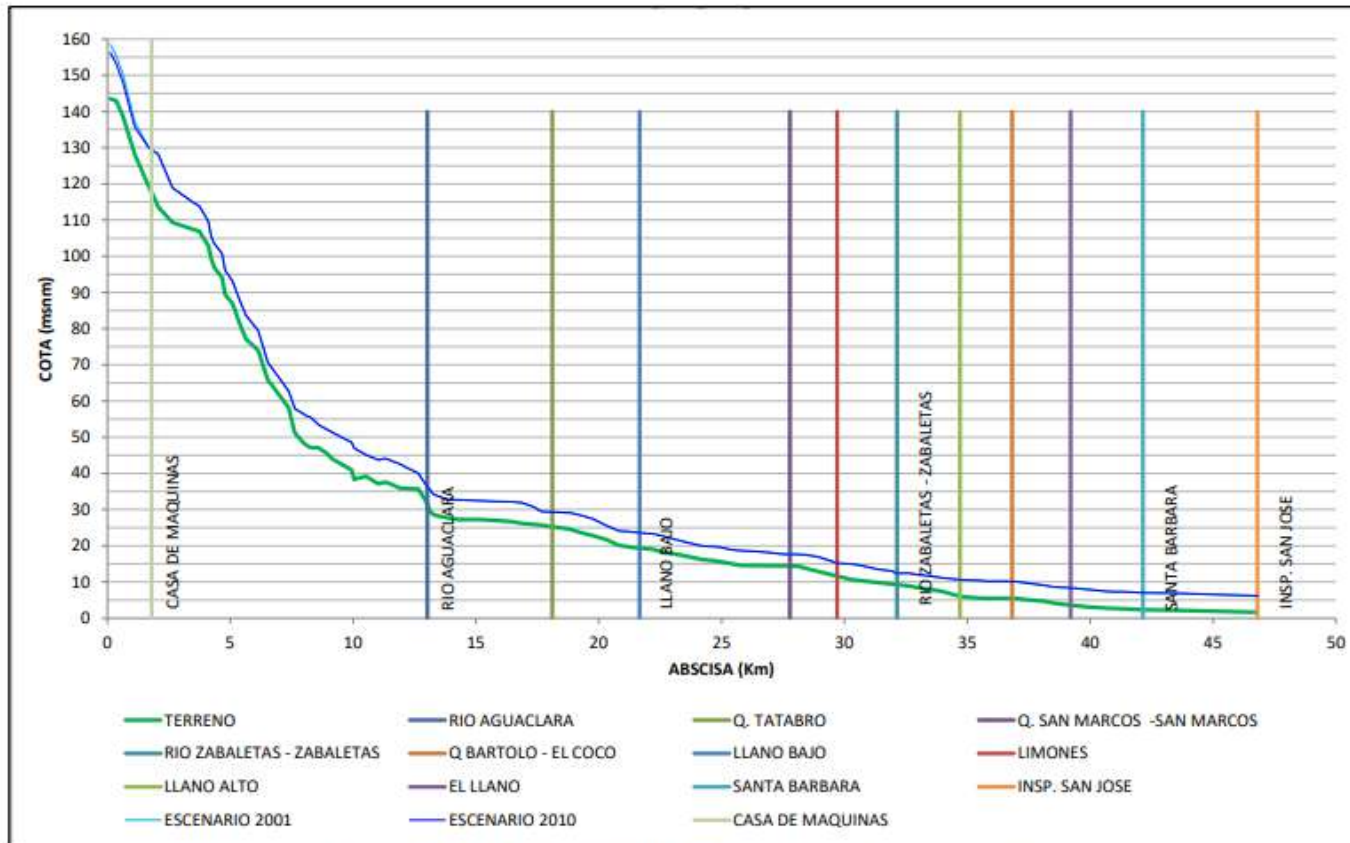
Figura 50. Perfil longitudinal y escenarios de inundación
