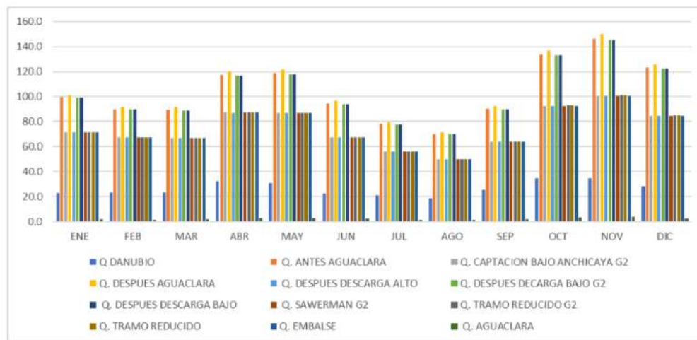
Figura 3 Caudales medios mensuales multianuales para las cuencas de estudio
