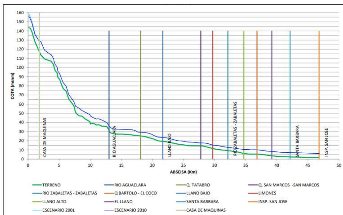
Figura 50. Perfil longitudinal y escenarios de inundación
