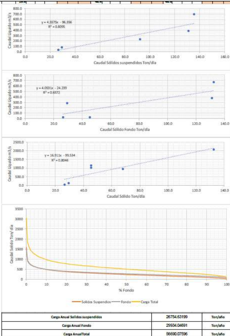
Figura 159. Transporte de Sedimentos, Estación antes descarga bajo campaña cero, uno, dos y tres. Fuente: Propia
