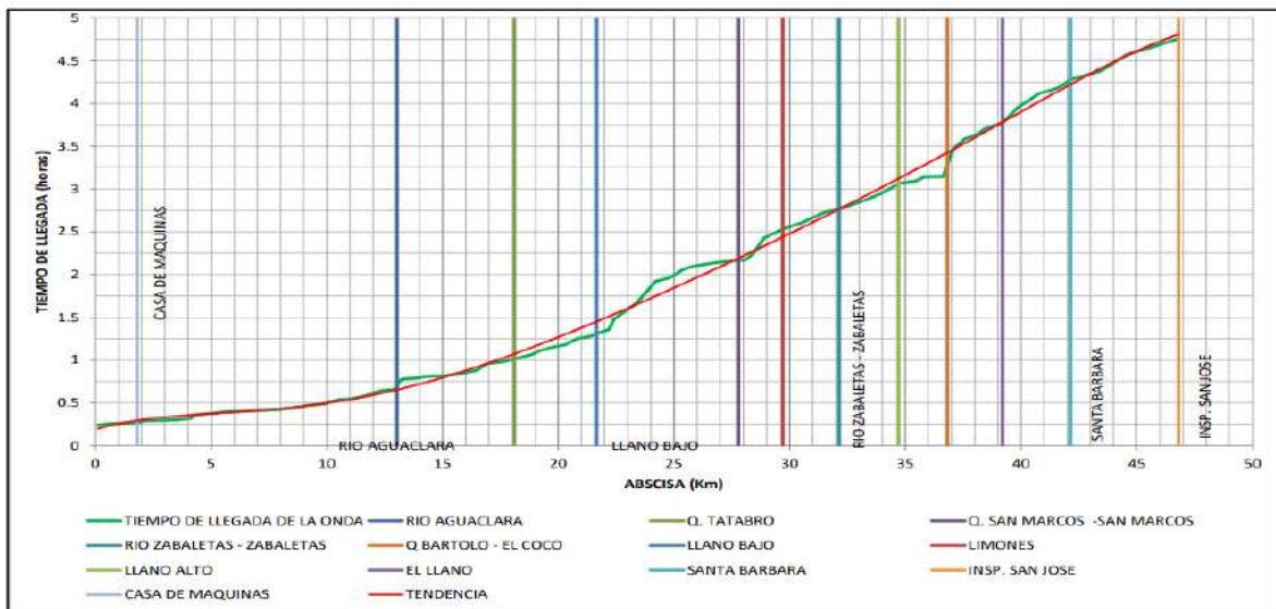
Figura 55. Tiempo de Llegada de Onda
