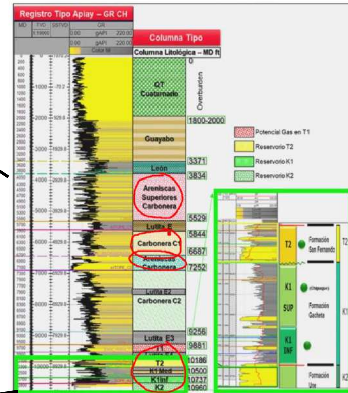
Figura 3 Columna estratigráfica generalizada de la cuenca de los Llanos Orientales (Llanos del Meta) y registro tipo para los reservorios en el Bloque Apiay
