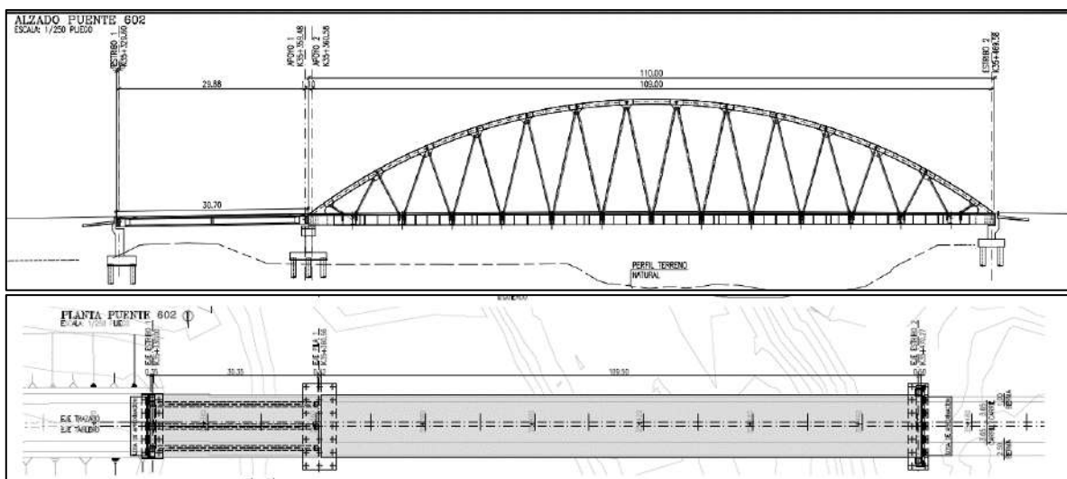
Figura 89 Esquema en perfil (arriba) y planta (abajo) del puente 602 - Río Bogotá sector Bosa Fuente: Información adicional con radicado 20246200426912 del 16 de abril de 2024 (Sociedad ALO Sur S.A.S., 2024)
