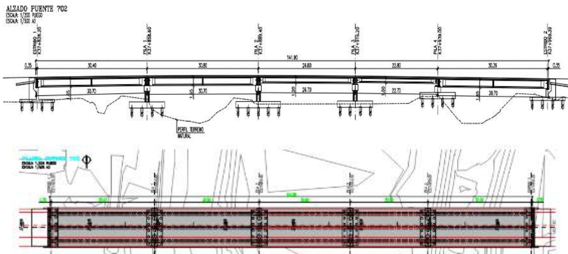
Figura 90 Esquema en perfil (arriba) y planta (abajo) del puente 702 – Río Balsillas occidental
