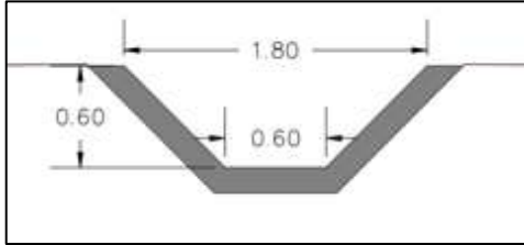
Figura 12 Sección típica canal longitudinal
