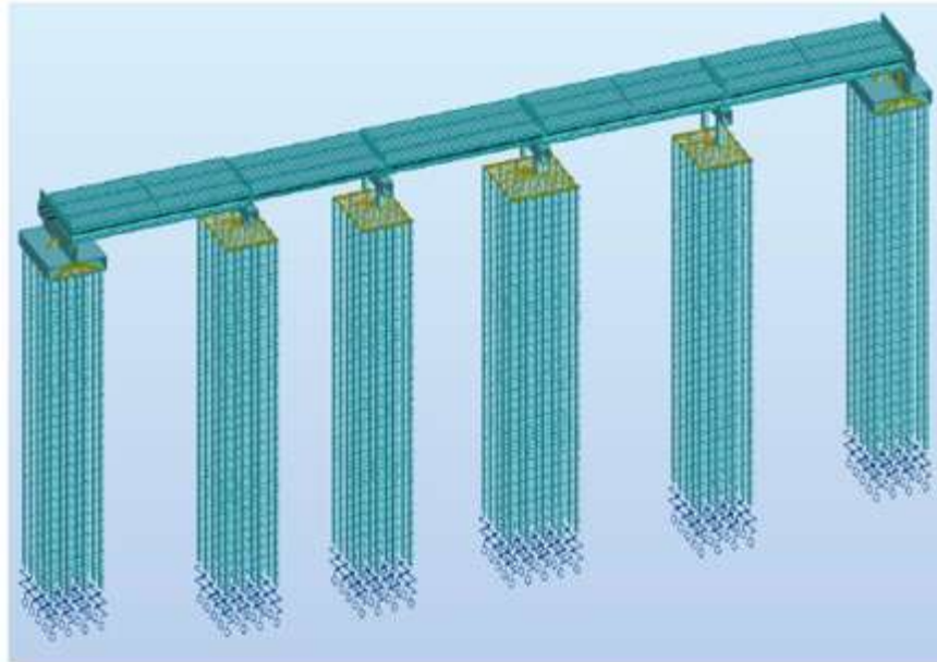
Figura 9 Modelo estructural puente 702 Fuente: Radicado 20246200426912 del 16 /04/2024
