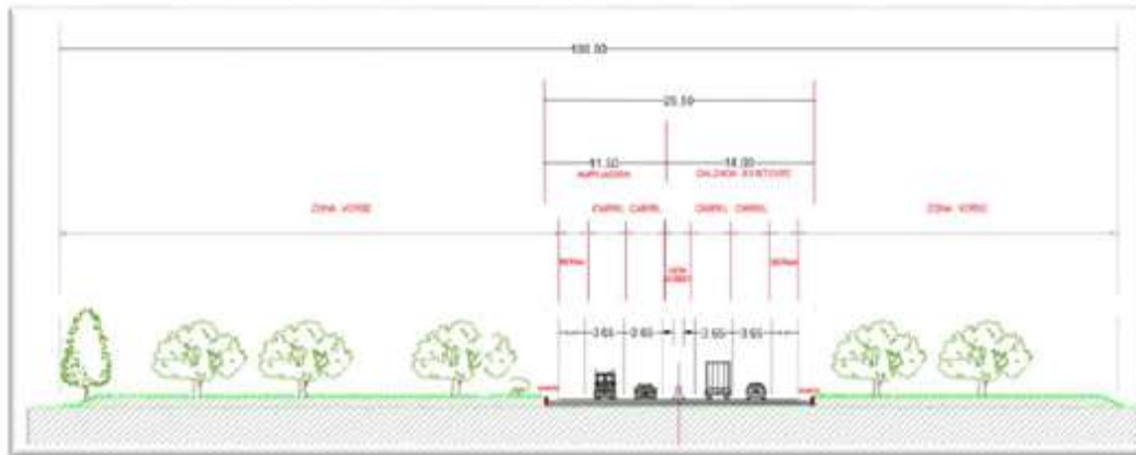
Figura 4. Sección típica transversal UF6 Fuente: Radicado 20246200426912 del 16 /04/2024
