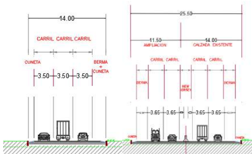
Figura 88 Sección transversal actual (izquierda) vs sección transversal proyectada con doble calzada (derecha)
