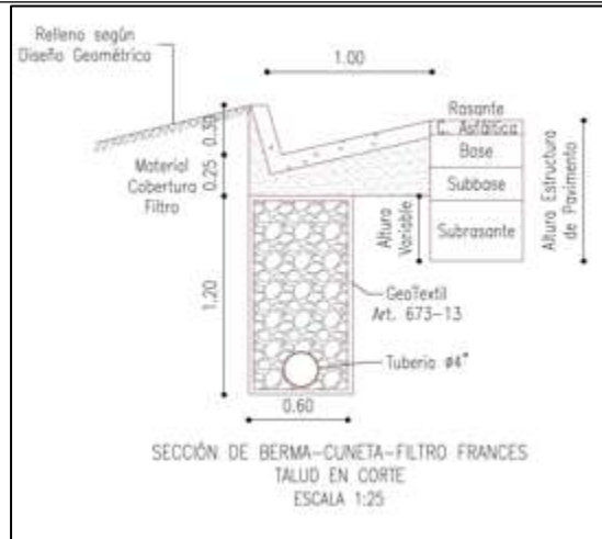
Figura 126 Sección típica cuneta
