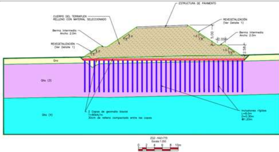
Figura 131 Sección transversal talud de relleno K42+770 Fuente: Radicado 20246200426912 del 16 /04/2024
