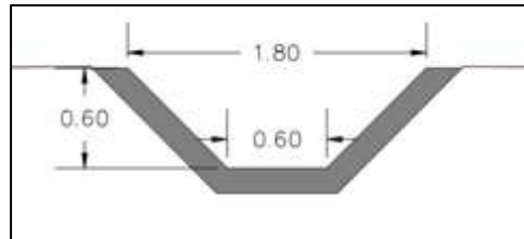
Figura 127 Sección típica canal longitudinal
