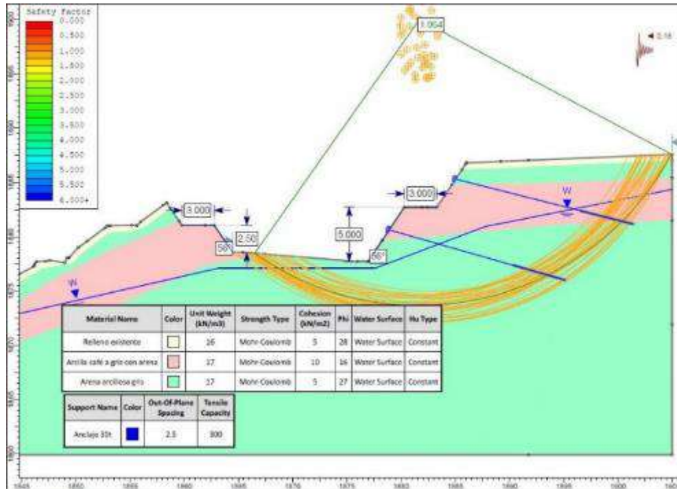
Figura 85 Análisis de equilibrio límite pseudo-estático para el corte del K49+300. F_s=1,064
