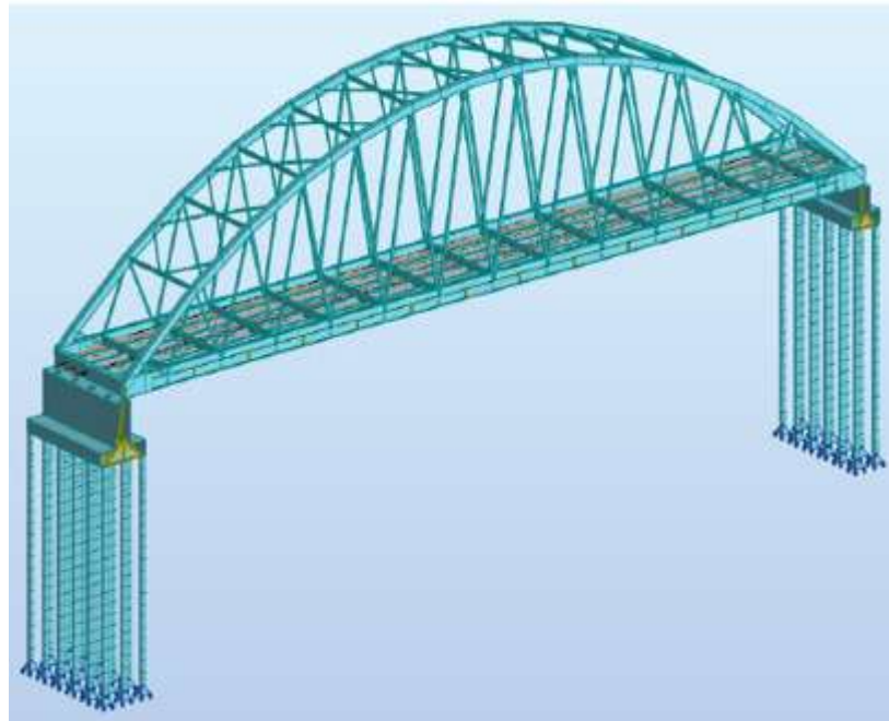
Figura 8 Modelo estructural puente 602 Fuente: Radicado 20246200426912 del 16 /04/2024
