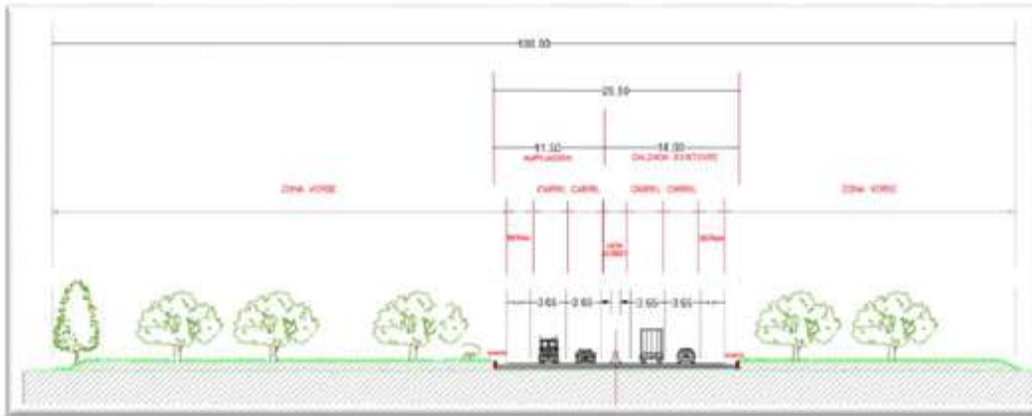
Figura 122. Sección típica transversal UF6
