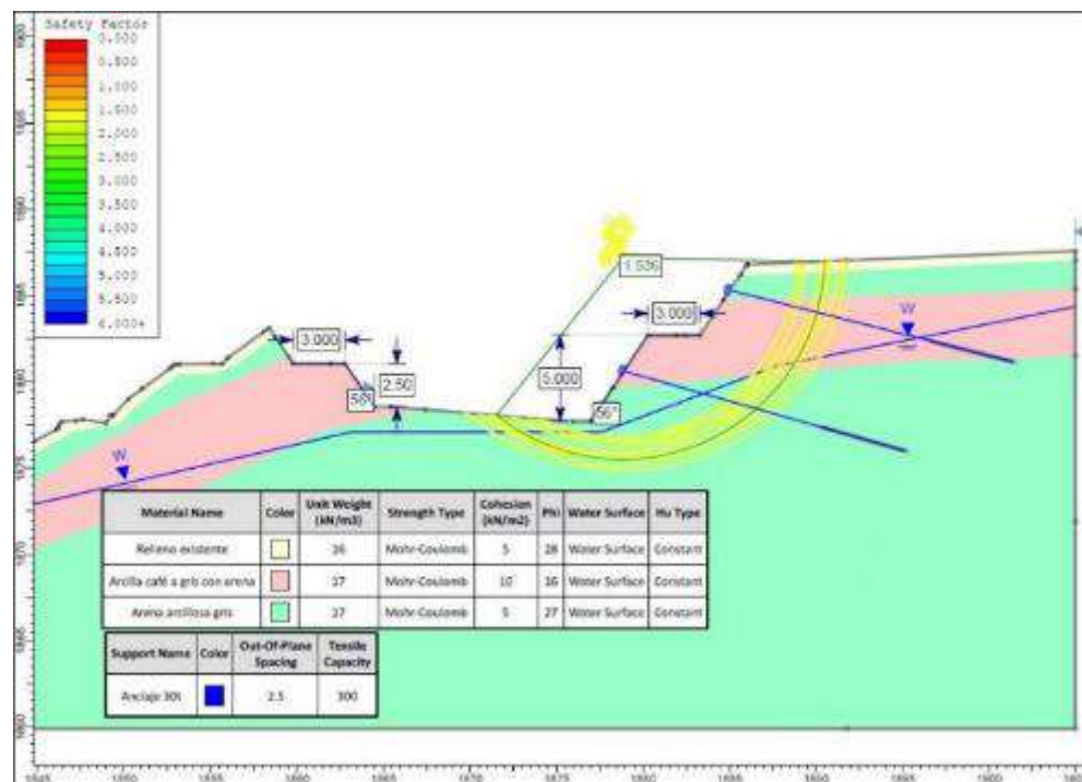
Figura 84 Análisis de equilibrio límite estático para el corte del K49+300. F_s=1,536 Fuente: Información adicional con radicado 20246200426912 del 16/04/2024 (Sociedad ALO Sur S.A.S., 2024)
