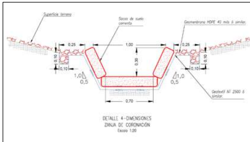
Figura 15 Sección típica zanja de coronación
