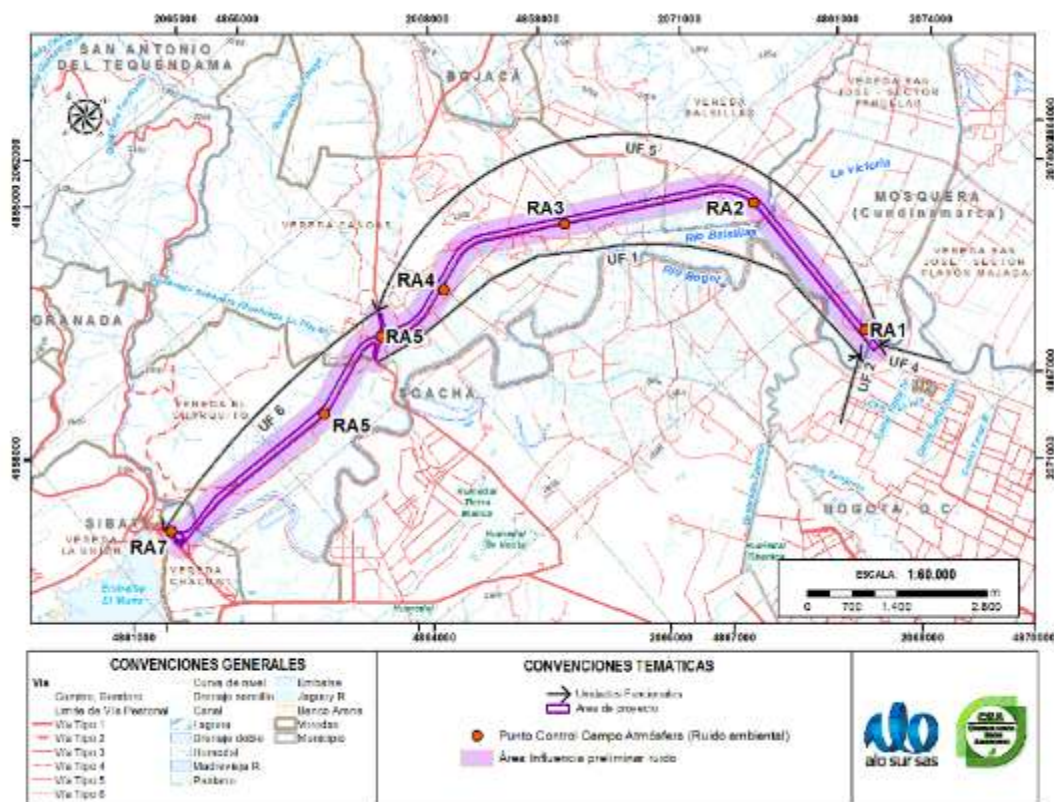
Figura 49 Puntos de monitoreo ruido ambiental
