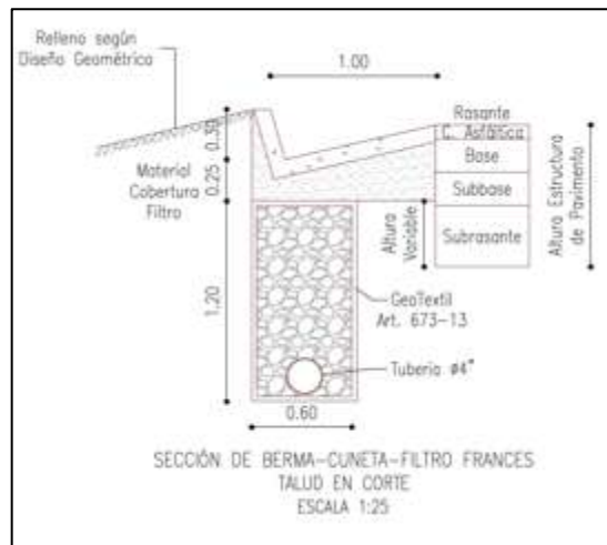
Figura 11 Sección típica cuneta
