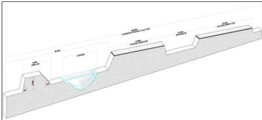
Figura 18 Esquema en sección transversal de la localización del Jarillón dentro del corredor
