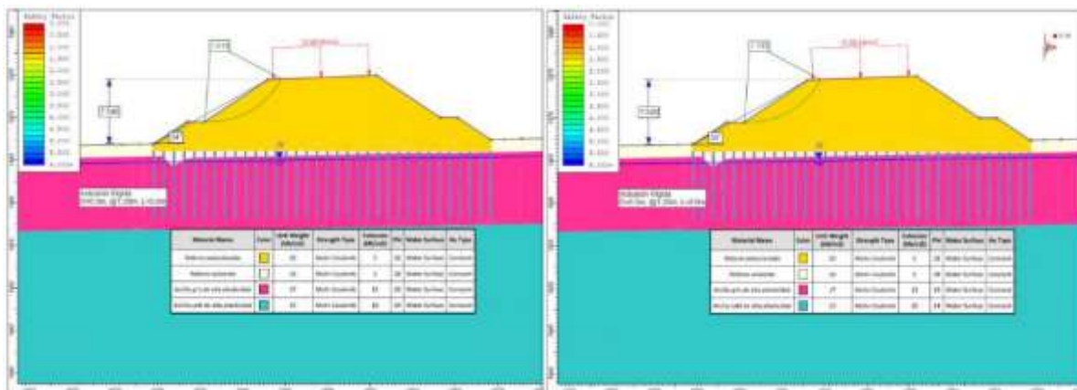
Figura 86 Análisis de equilibrio límite para terraplén del K42+770. F.S\ est=1,614 - F.S\ seudo=1,189
