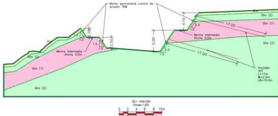
Figura 132 Sección transversal talud de corte K49+300 Fuente: Radicado 20246200426912 del 16 /04/2024
