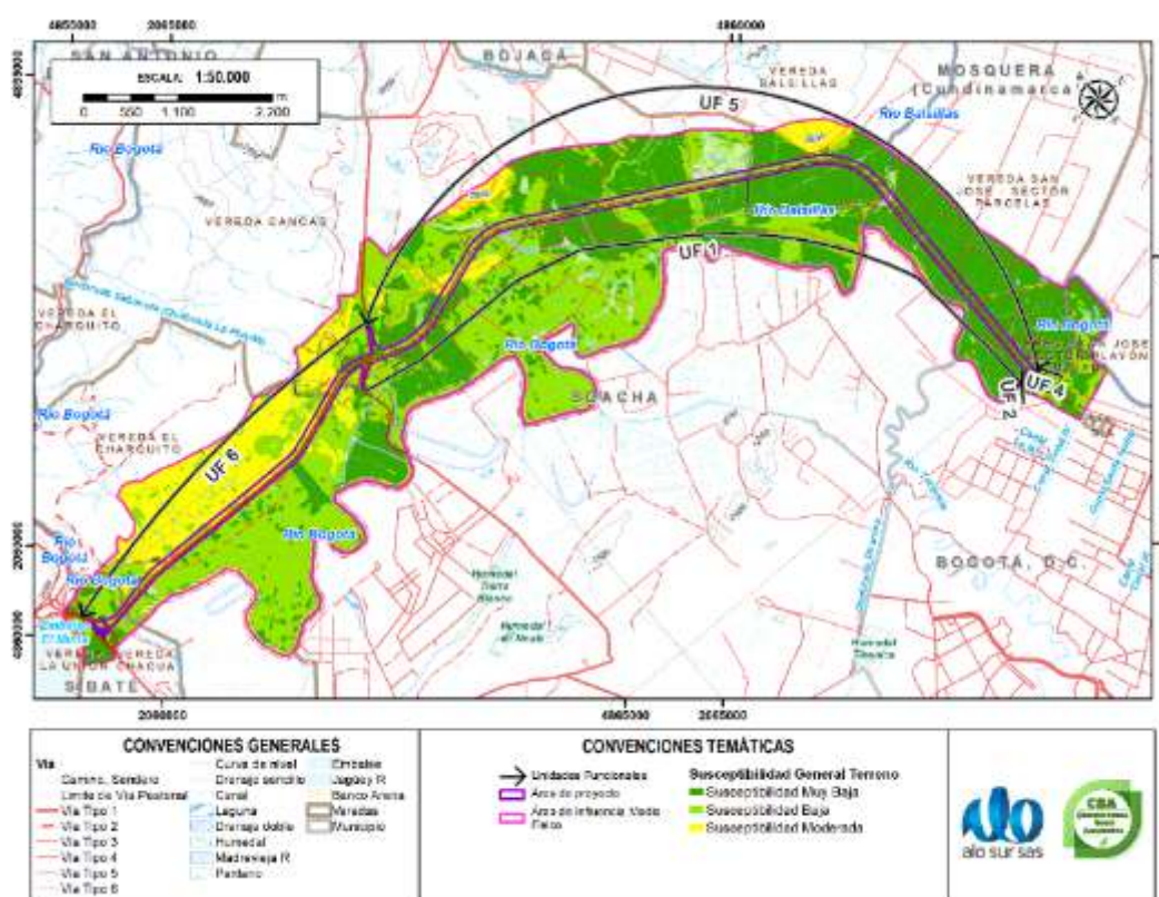
Figura 44 Susceptibilidad general del terreno (SGT) del área de influencia propuesta Fuente: Información adicional con radicado 20246200426912 del 16/04/2024 (Sociedad ALO Sur S.A.S., 2024)
