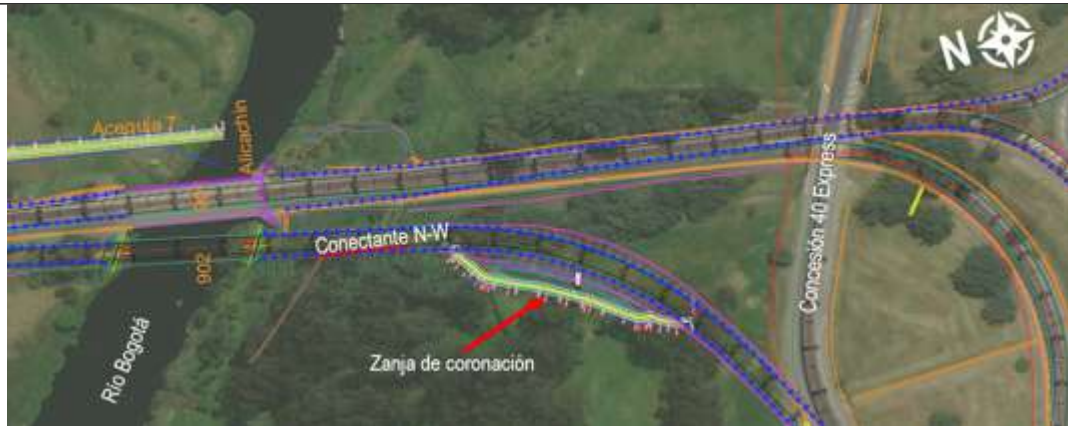
Figura 14 Esquema en planta zanja de coronación en conectante Chusacá
