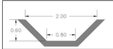
Figura 128 Sección típica acequia
