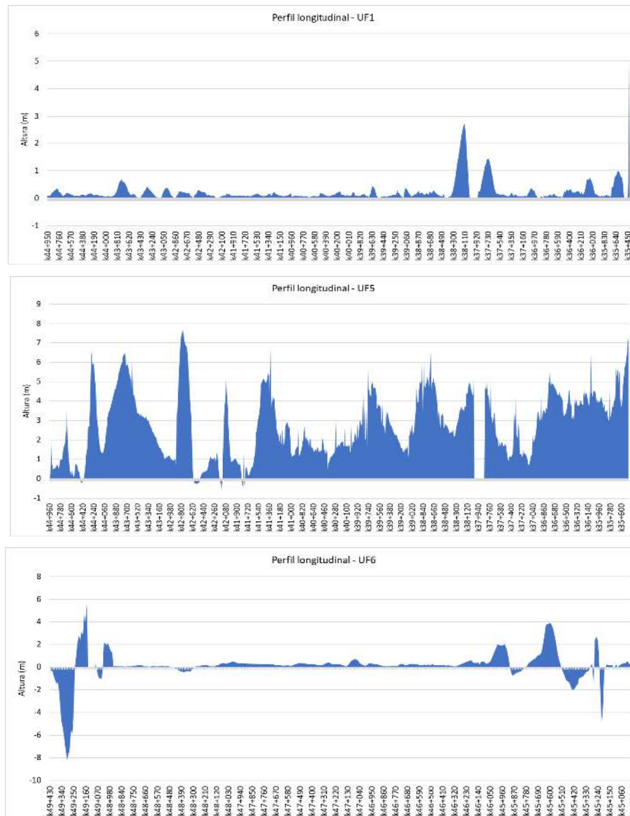
Figura 83 Perfil longitudinal del movimiento de tierras (rellenos y cortes) por unidad funcional y según abscisado
