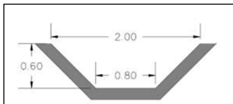
Figura 13 Sección típica acequia
