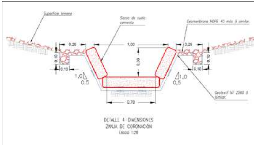
Figura 130 Sección típica zanja de coronación
