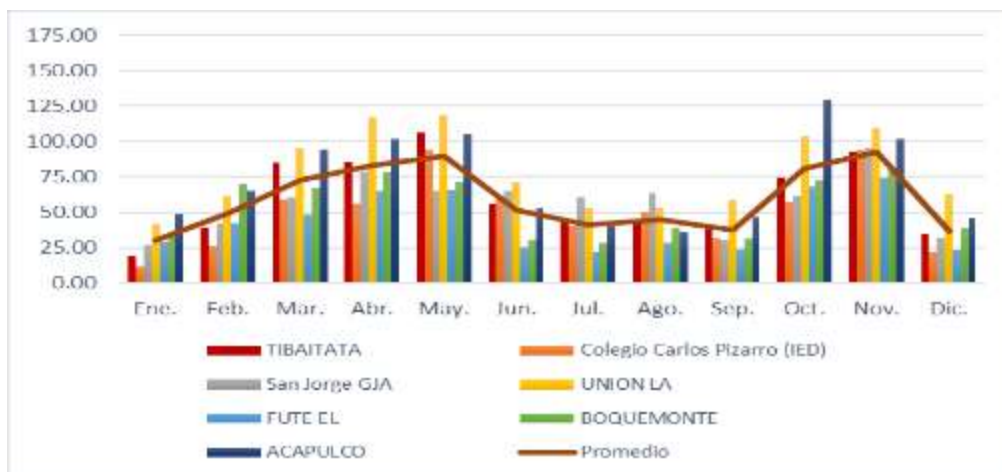
Figura 46 Histograma de precipitación mensual multianual de estaciones analizadas
