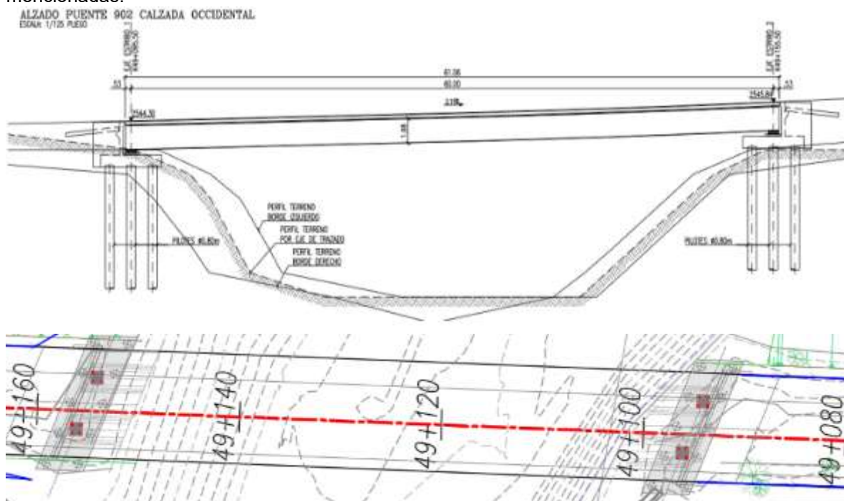
Figura 91 Esquema en perfil (arriba) y planta (abajo) del puente 902 – Río Bogotá Alicachín
