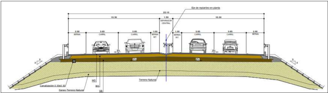
Sección transversal tipo UF 8
