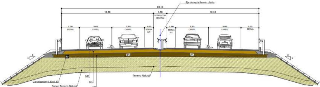
Figura 1 Sección transversal tipo UF 8
