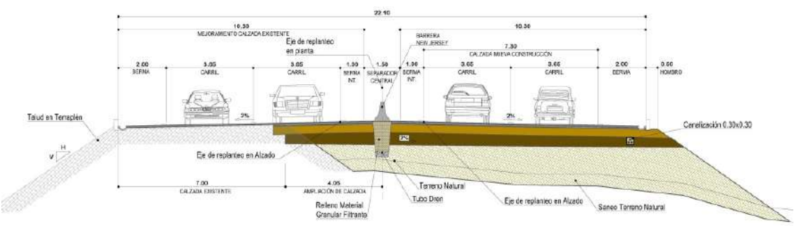
Sección transversal tipo UF 9
