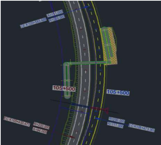
Figura 7 Diseño tipo puente peatonal
