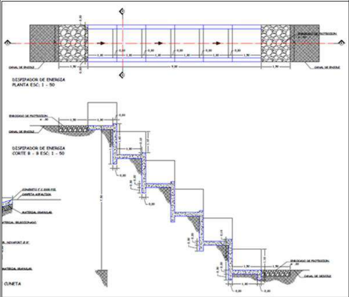
Figura 8 Diseño tipo de disipador de energía
