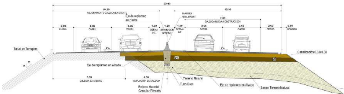
Figura 2 Sección transversal tipo UF 9
