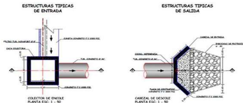
Figura 6 Diseño tipo de alcantarillas
