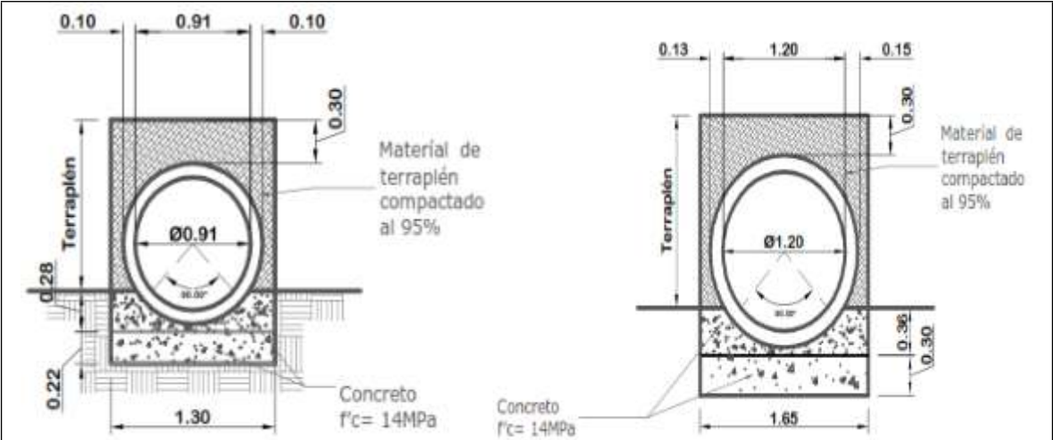
Figura 7 Diseño tipo de alcantarillas
