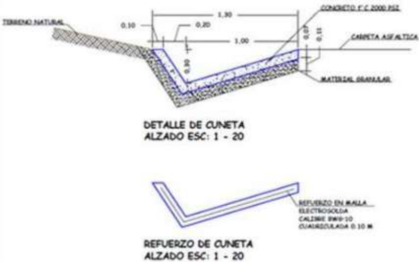
Figura 6 Diseño tipo de cunetas triangular
