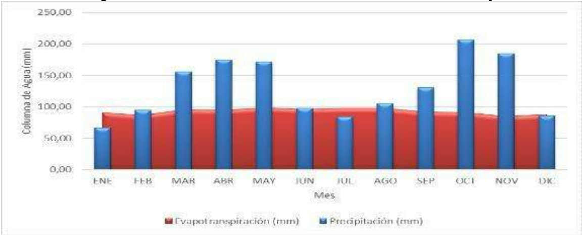
Figura 18 Balance hidroclimático área de influencia unidades funcionales 8 y 9.
