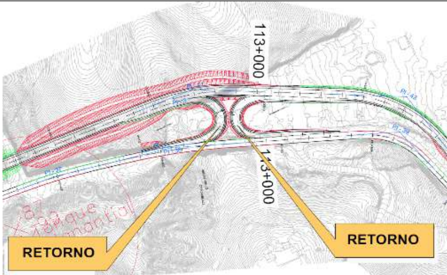
Figura 4 Diseño tipo para los retornos
