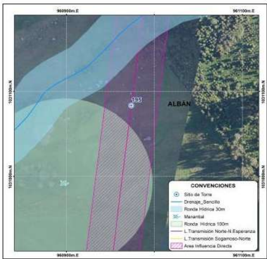
Figura 19. Sitio de Torre 195 línea de transmisión Norte – Nueva Esperanza Fuente: Ortofotos LIDAR 2015 extraídas de ARCGIS
