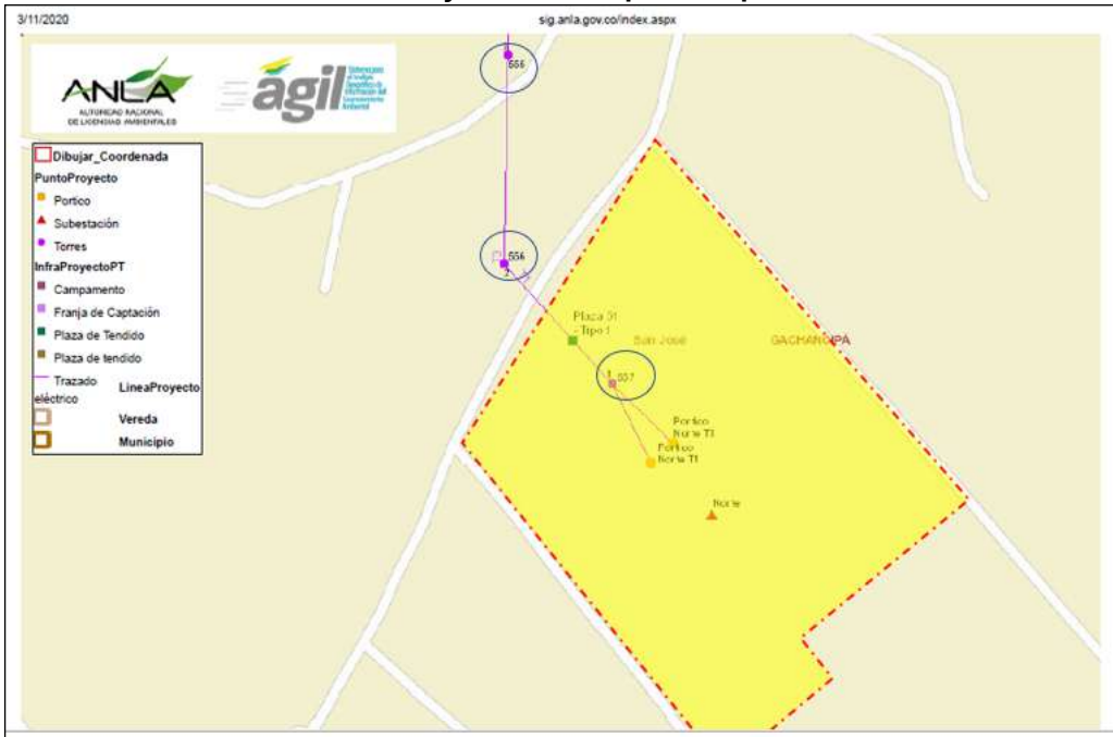
Figura 47 Ubicación torres 555, 556 y 557 con respecto al predio de la Subestación Norte
