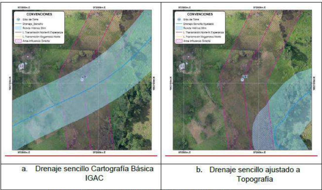
Figura 8. Sitio de Torre 287 línea de transmisión Norte – Nueva Esperanza Fuente: Ortofotos LIDAR 2015 extraídas de ARCGIS
