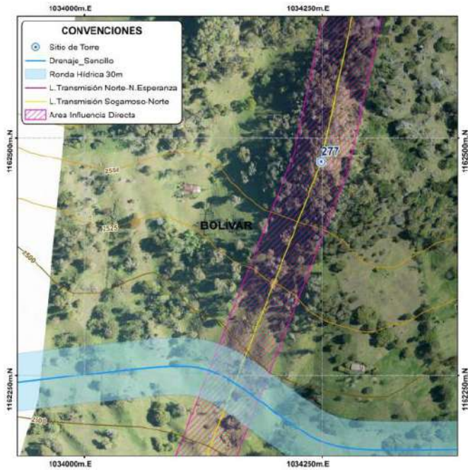
Figura 31. Sitio de Torre 277 línea de transmisión Sogamoso – Norte Fuente: Ortofotos LIDAR 2015 extraídas de ARCGIS
