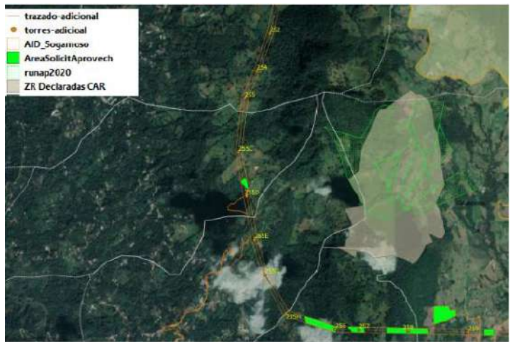
Figura 60. Vano Torres 259-252
