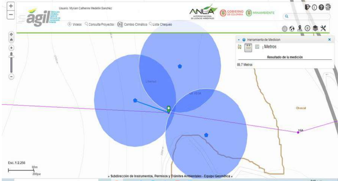
Figura 23 Distancia de la Torre 161 al manantial más cercano del área de influencia
