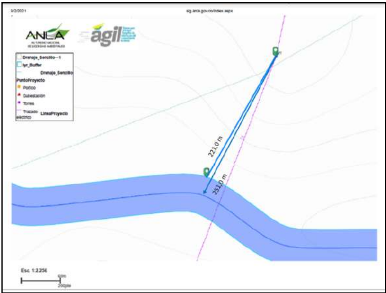
Figura 7 Distancia de la Torre 277 al drenaje sencillo
