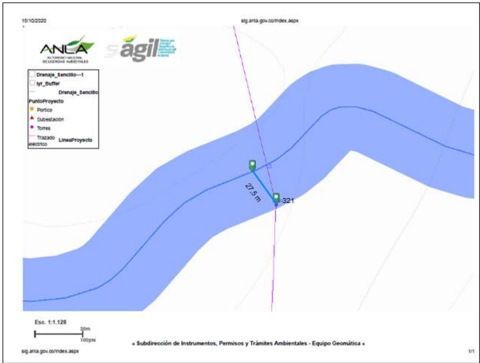
Figura 8 Distancia de la Torre 321 al drenaje sencillo
