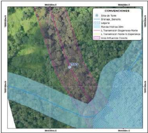
Figura 14. Sitio de Torre 255G línea de transmisión Norte – Nueva Esperanza Fuente: Ortofotos LIDAR 2015 extraídas de ARCGIS
