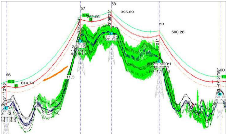
Figura 67. Perfil de vegetación torres 56 - 60 Fuente: GEB, 2020
