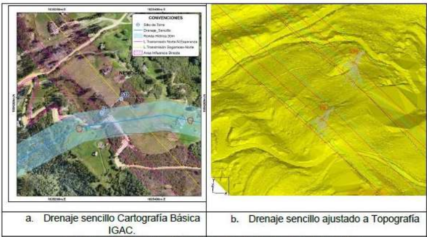
Figura 22. Sitio de Torre 19 línea de transmisión Norte – Nueva Esperanza Fuente: Ortofotos LIDAR 2015 extraídas de ARCGIS
