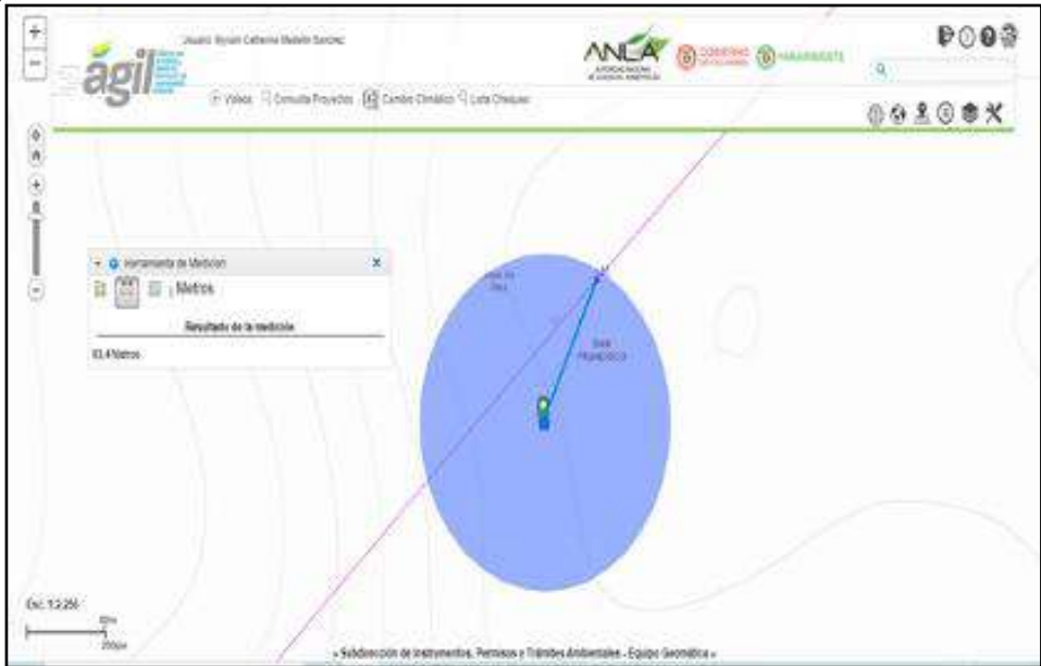
Figura 21 Distancia de la Torre 152 al manantial más cercano del área de influencia
