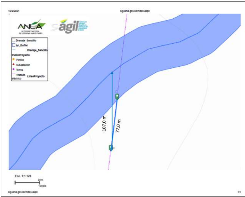
Figura 12 Distancia de la Torre 195 al drenaje sencillo
