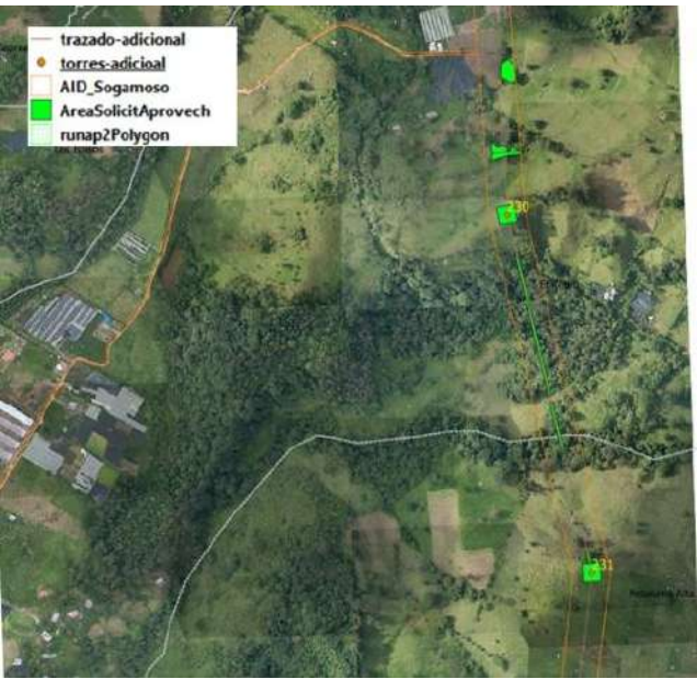
Figura 61. Vano Torres 230-231 Fuente: GEB – Imagen LIDAR 2015
