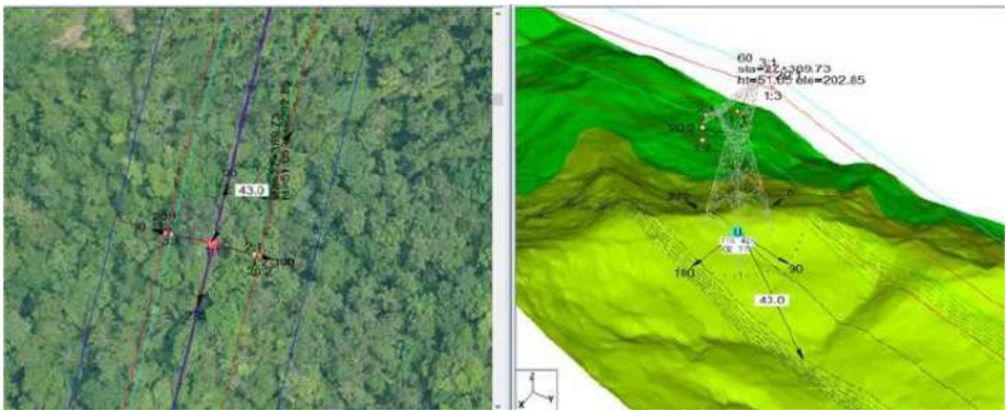
Figura 36. Vista en planta sitio de Torre 60 línea de transmisión Sogamoso – Norte Fuente: Ortofotos LIDAR 2015 extraídas de PLS-CADD
