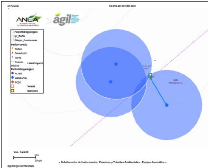
Figura 20 Distancia de la Torre 151 al manantial más cercano del área de influencia
