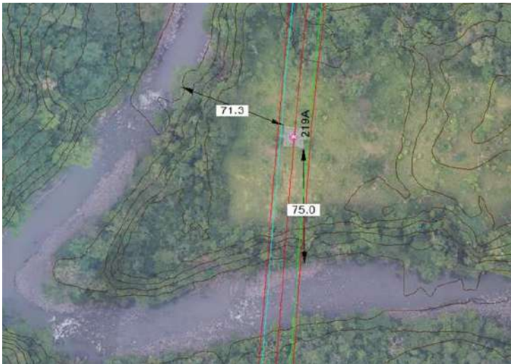
Figura 34. Vista en planta Sitio de Torre 219 línea de transmisión Sogamoso – Norte Fuente: Ortofotos LIDAR 2015 extraídas de PLS-CADD
