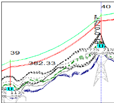
Figura 63. Perfil de vegetación torres 39-40 Fuente: GEB, 2020
