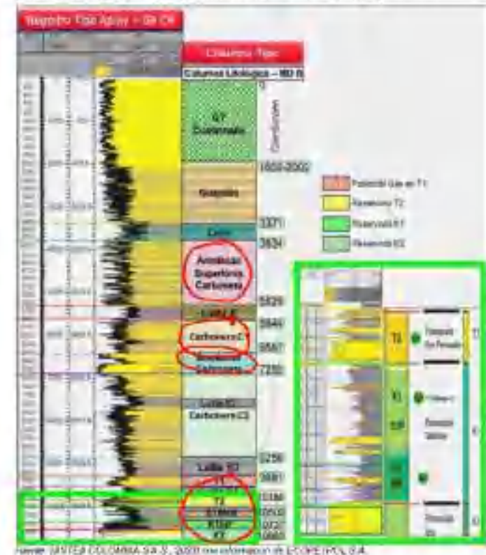
Figura 3 Columna estratigráfica generalizada de la cuenca de los Llanos Orientales (Llanos del Meta) y registro tipo para los reservorios en el Bloque Apurí
