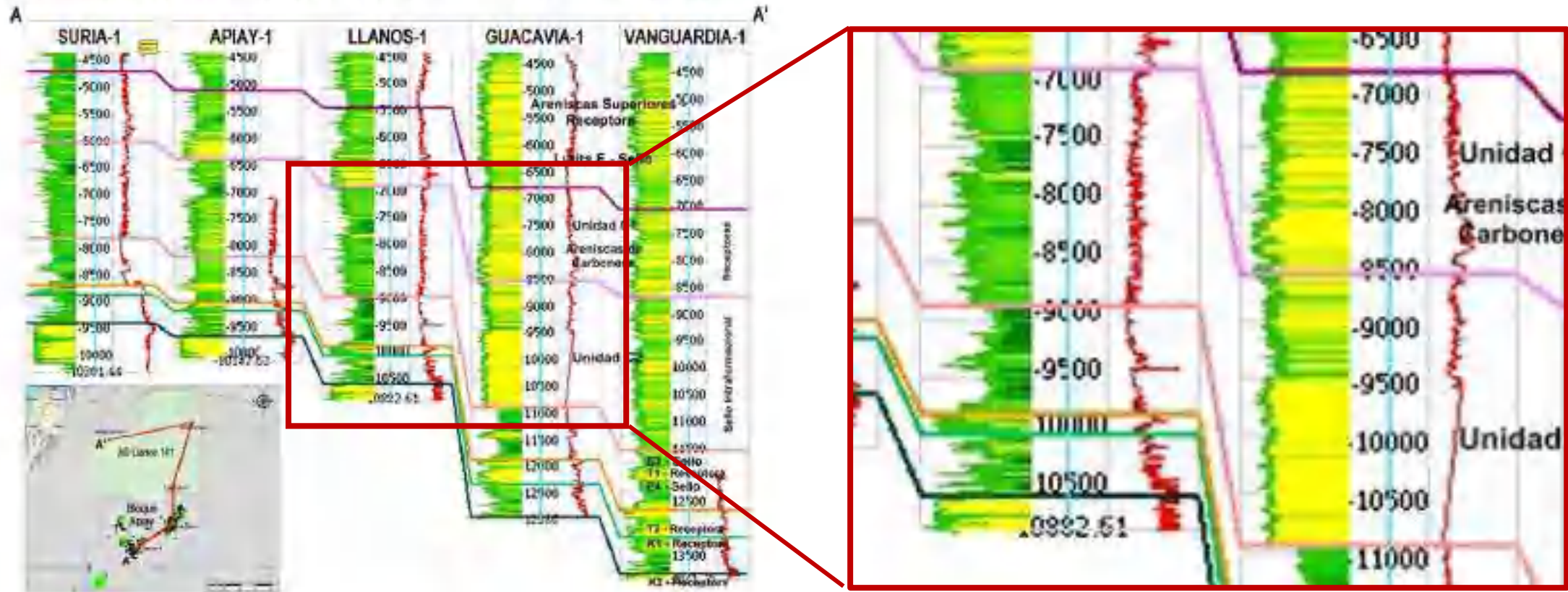
Correlación estratigráfica pozos Suria-1, Apiay-1 y prospectos Llanos-1, Guacavía-1 y Vanguardia-1
