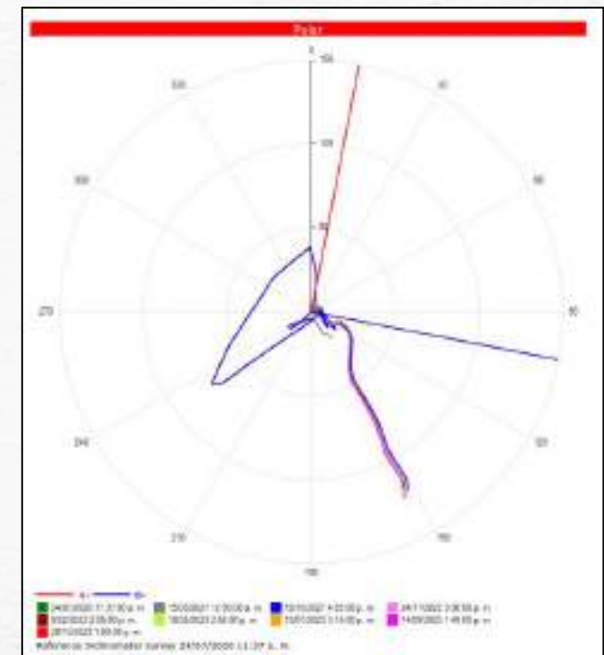
Graficas de lecturas de orientación de los desplazamientos medidos por el inclinómetro
