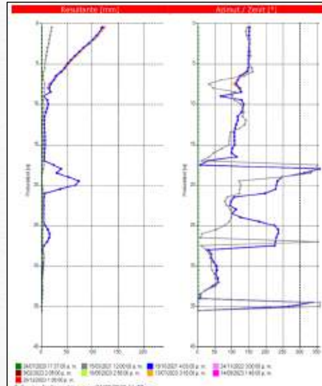
Graficas de lecturas de desplazamientos del inclinómetro
